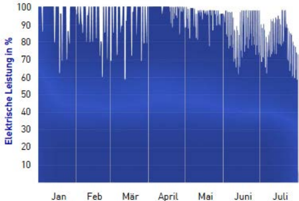
Leistungsdiagramm einer kerntechnischen Anlage im Lastfolgebetrieb
