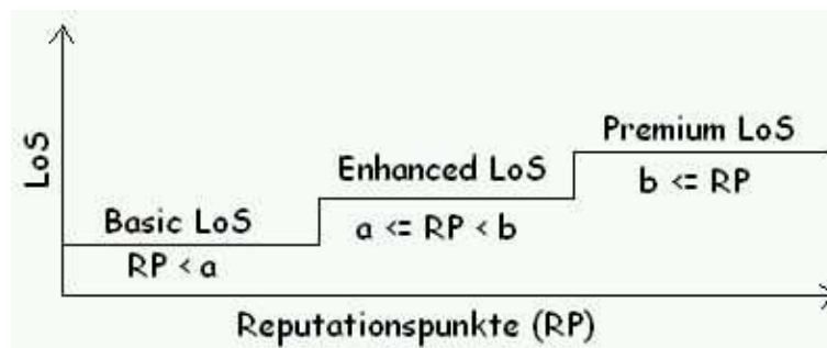
Abbildung 4.3: Servicelevel [3, S. 2]
