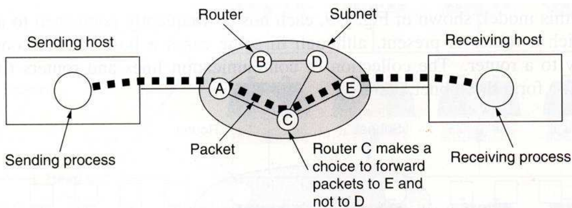
Abbildung 1.16: WAN [tanen2]
