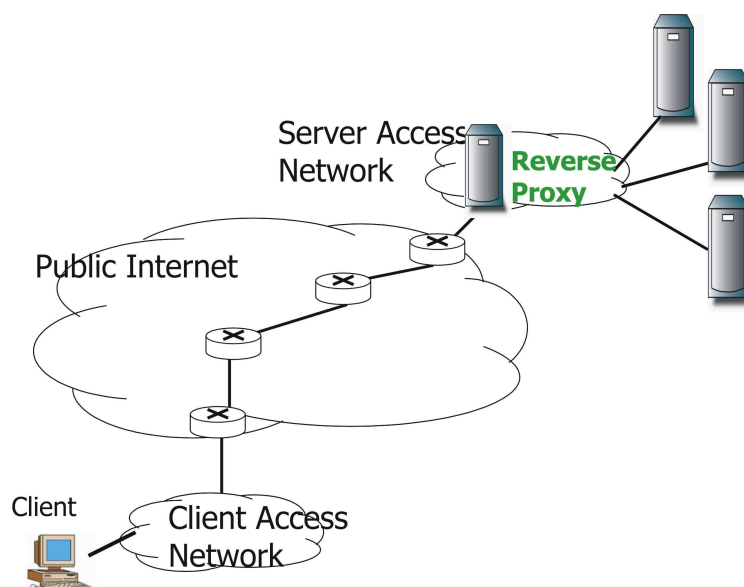
Abbildung 6.4: Reverse Proxy
