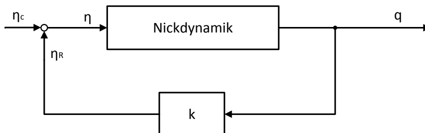
Abbildung 2: Nickdämpfer-Schaltung
