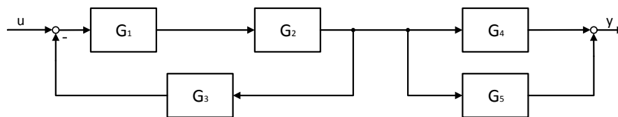
Abbildung 1: Blockschaltbild
