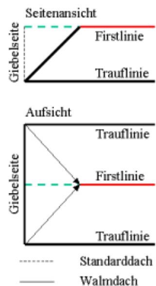
Abb. 65: Bildung eines Walmdaches
