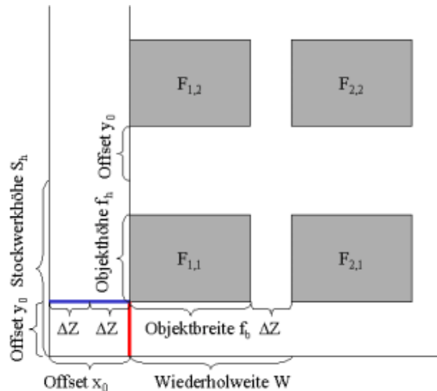
Abb. 80: Parameter für Verteilung von Fenstern
