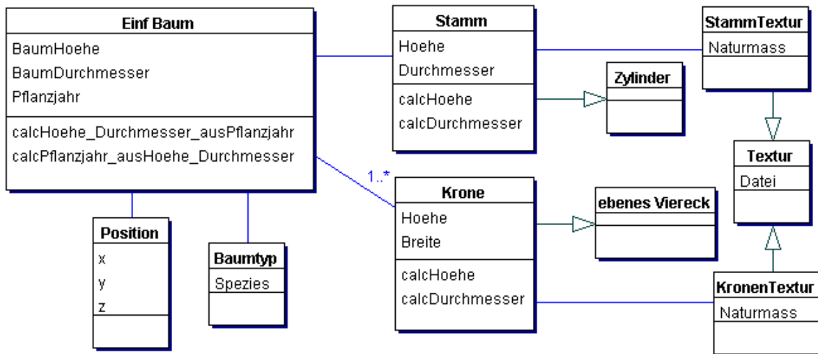
Modell 4: Struktur des Kreuztexturmodells
