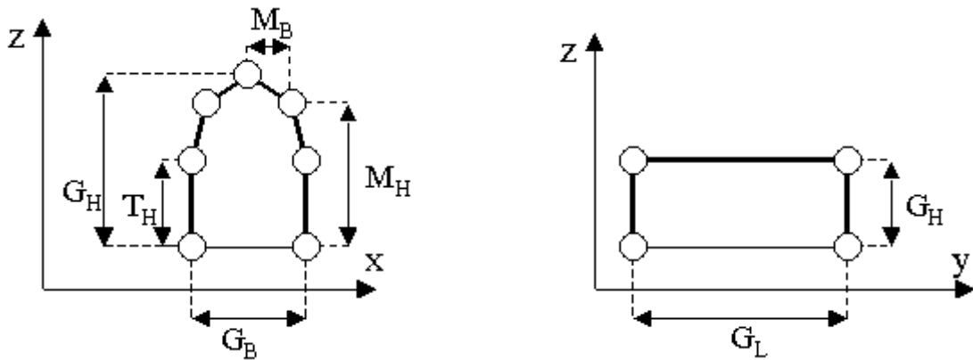
Abb. 57: Maße des Mauerwerks
