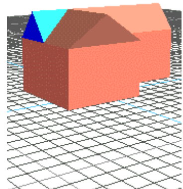
Abb. 53: Komplex aggregiertes Gebäude nach der Anwendung des und-Operators
