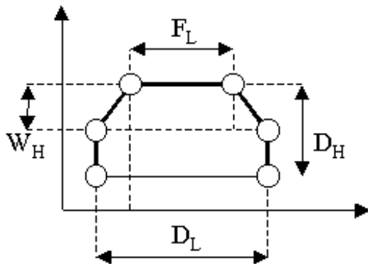
Abb. 71: Parameter im Dachlängsschnitt: Dachlänge D_L - Firstlänge F_L - Dachhöhe D_H - Walmhöhe W_H
