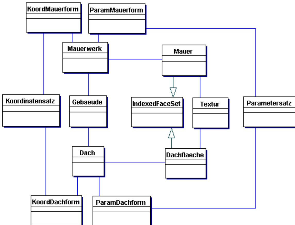
Modell 10: Modell für ein texturiertes Gebäude in Wandmodelltechnik
