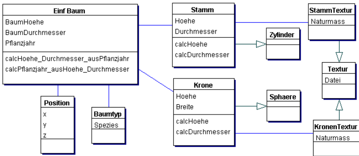
Modell 2: UML-Modell des Kugelbaummodells mit Textur
