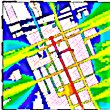
Abb. 4: Ergebnis einer Feldstärke-schätzung mittels Ray-Tracing
