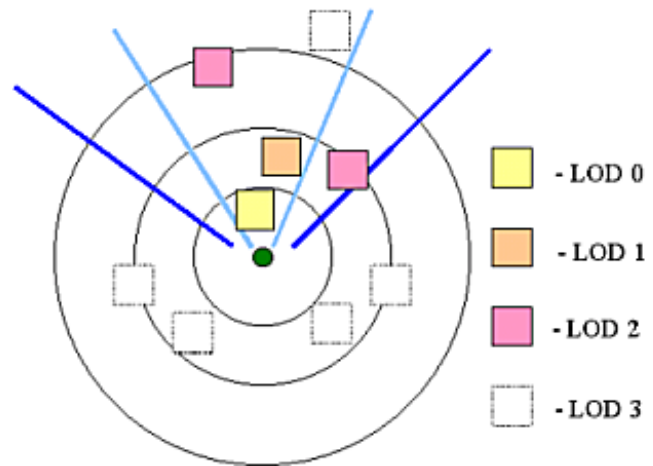
Abb. 28: LoD nach Entfernung-, Richtungs- und Sichtbarkeitsbedingungen
