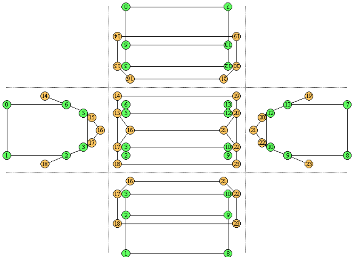
Abb. 86: Gemeinsame Punktstruktur von Mauerwerk und Dach
