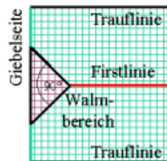
Abb. 68: Krüppelwalmdach in der Aufsicht
