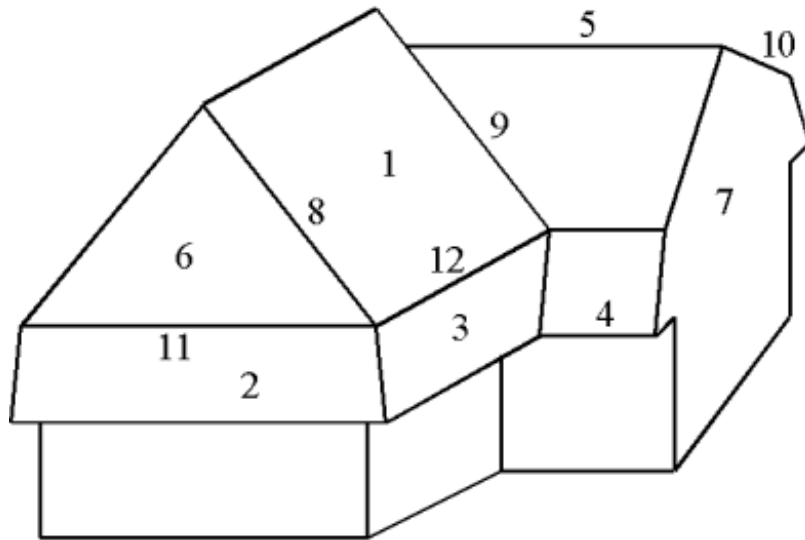
Abb. 60: Bezeichnungen von Dachelementen: 1 – Hauptdach, 2 – Mansarde-Walm, 3 – Mansarde, 4 – Traufe T, 5 – First F, 6 – Walm W, 7 – Giebel, 8 – Grat G, 9 – Kehle, 10 – Ortgang O, 11 – Walmbruch, 12 – Dachbruch Db
