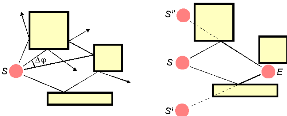
Abb. 3: Verfahren zur Funkraumberechnung: links Ray-Launching, rechts Ray Tracing
