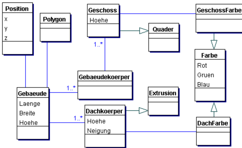
Modell 7: Einfaches Gebäudemodell in Volumenmodelltechnik
