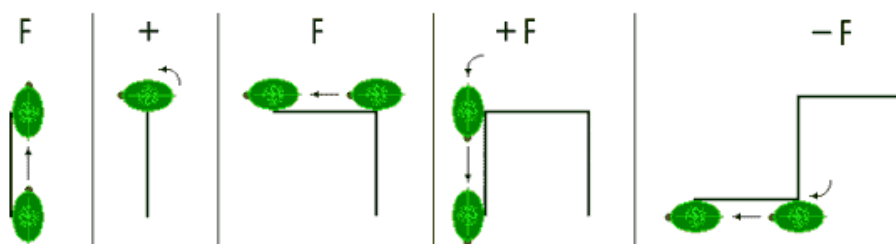
Abb. 35: Das Wort F+F+F-F ( \delta=90^\circ ) interpretiert durch den Igel
