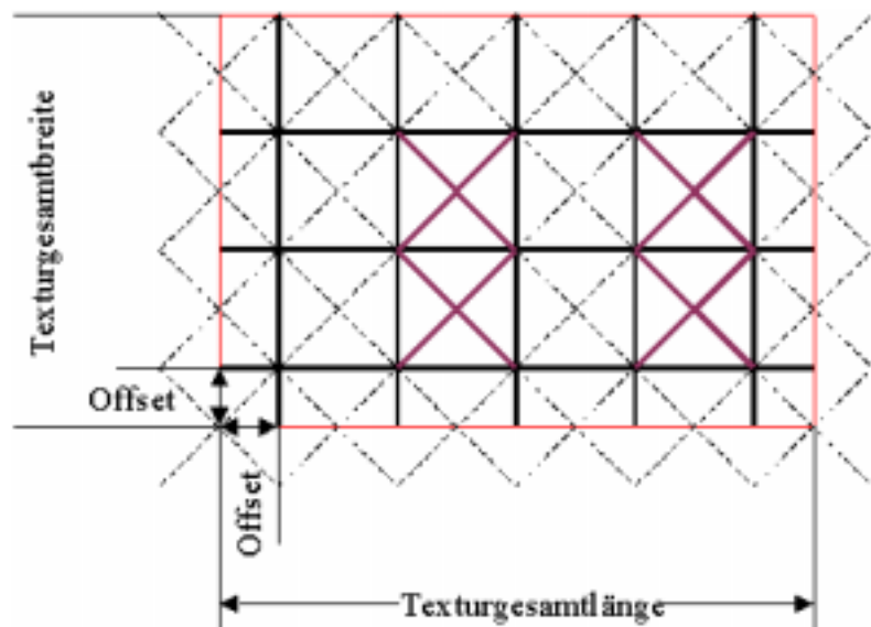
Abb. 77: Raster-Texturmodell
