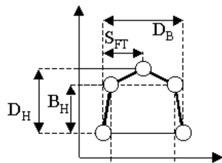
Parameter Dachquerschnitt: Dachhöhe D_H - Dachbruchweite D_B - Höhe Dachbruch B_H - Dachbreite D_B - Abstand First Traufe S_{FT}
