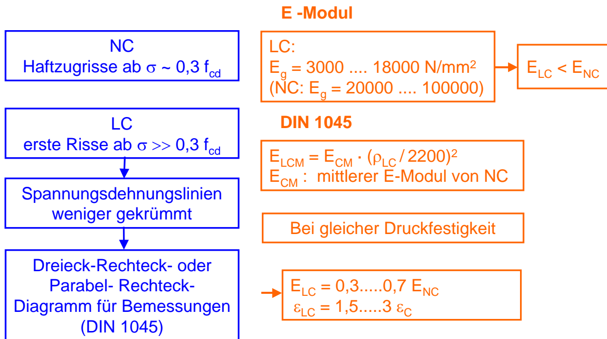
Bild 14: Formänderungen von Leichtbeton
